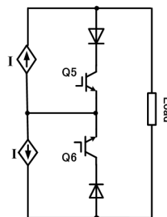
Fig. 2. Two-level CSI module
